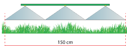
SCHÉMA DE PULVÉRISATION AVEC BUSES DE SÉRIE
